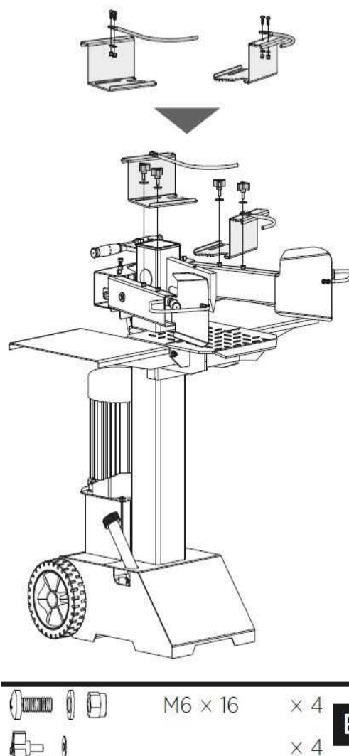
Abb. 11: Montage Steuerhebel
