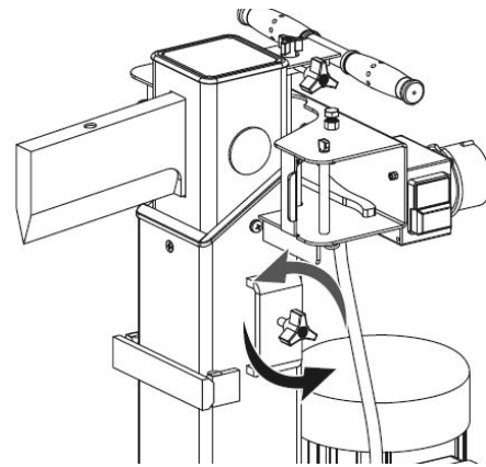
Abb. 7: Montage Auflagetisch
