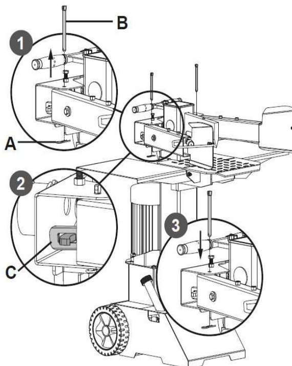
Abb. 10: Montage Bedienarme
