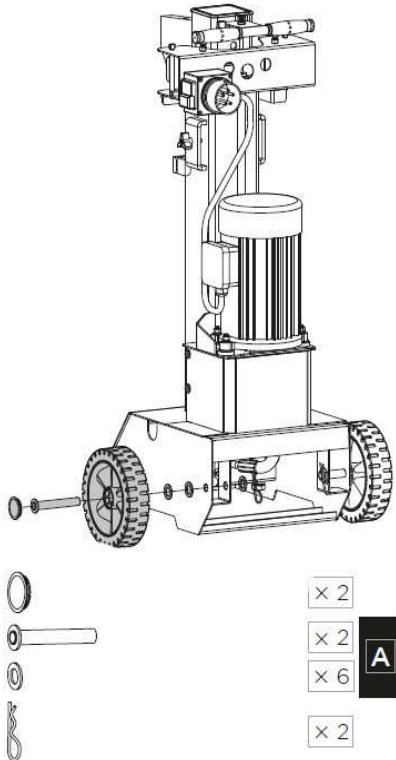
Abb. 6: Radmontage
