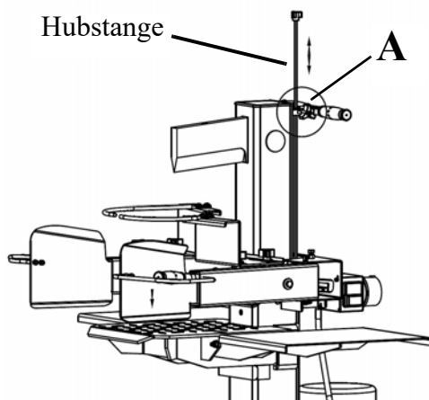
Abb. 12: Keilhub
