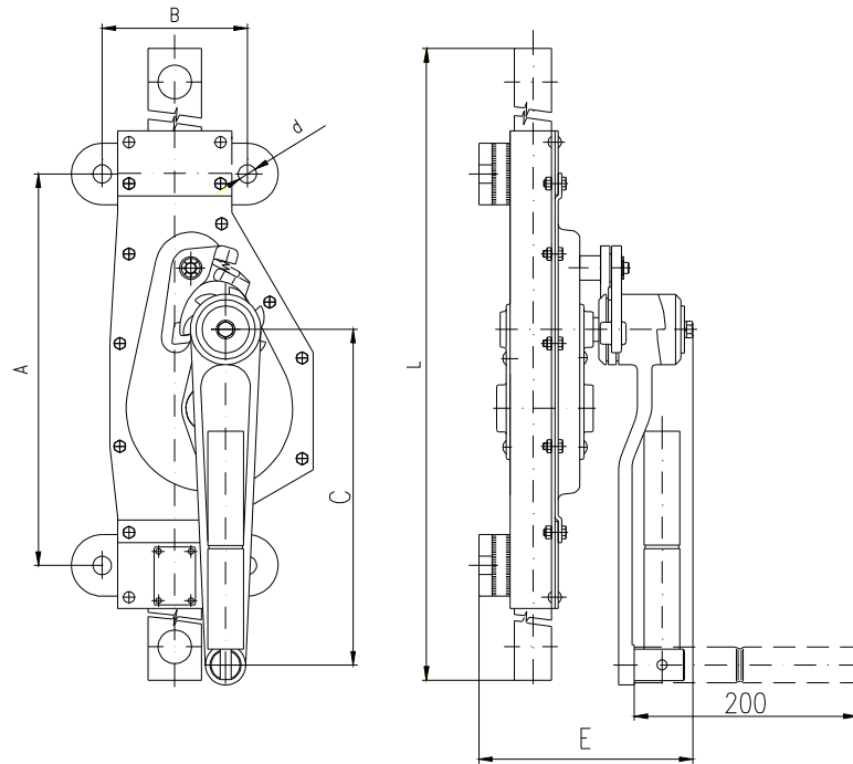
Abb.1 Heber Typ 15-00 CON - W
